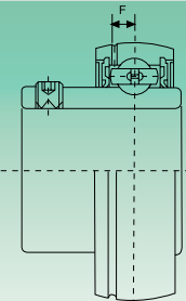
SB 2S anello esterno cilindrico, con gola di lubrificazione outer cylindrical ring, with relubrication groove
